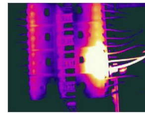
Pregretje elektronike
